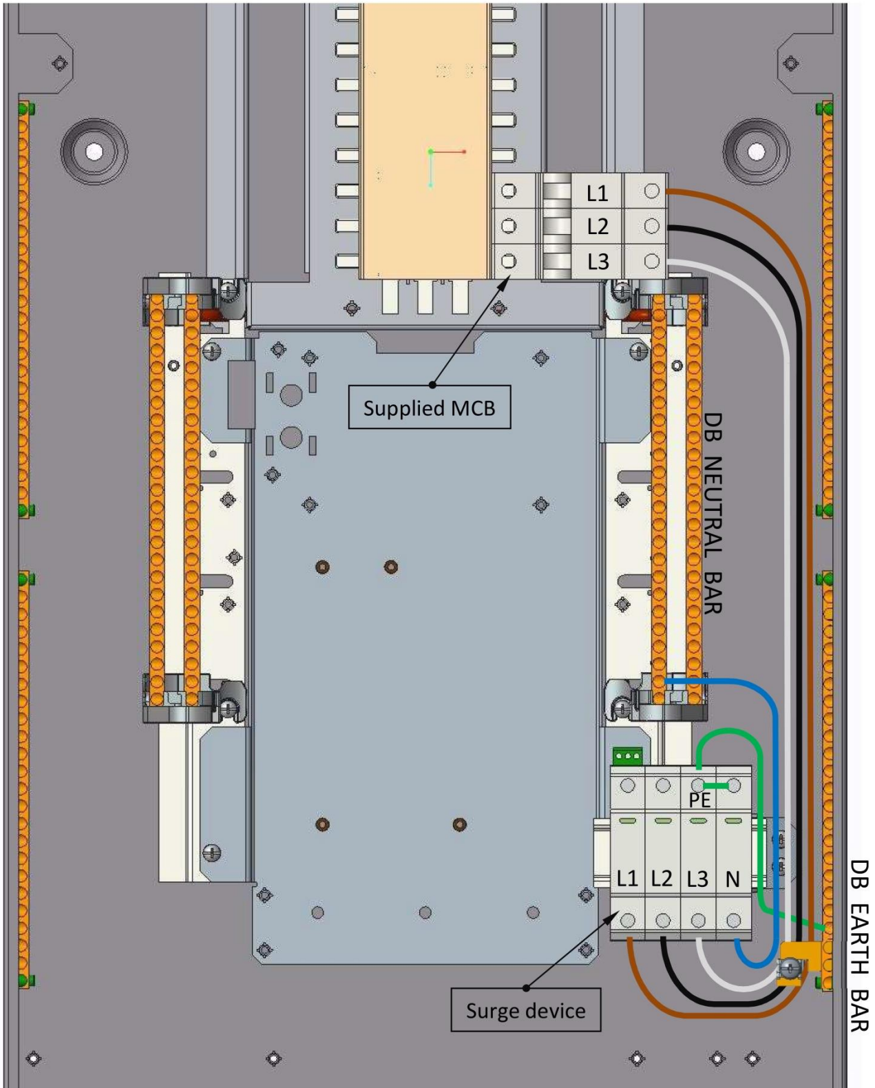
Wiring Diagram - Fig. 2
